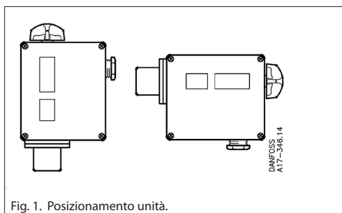
Fig. 1. Posizionamento unità.
